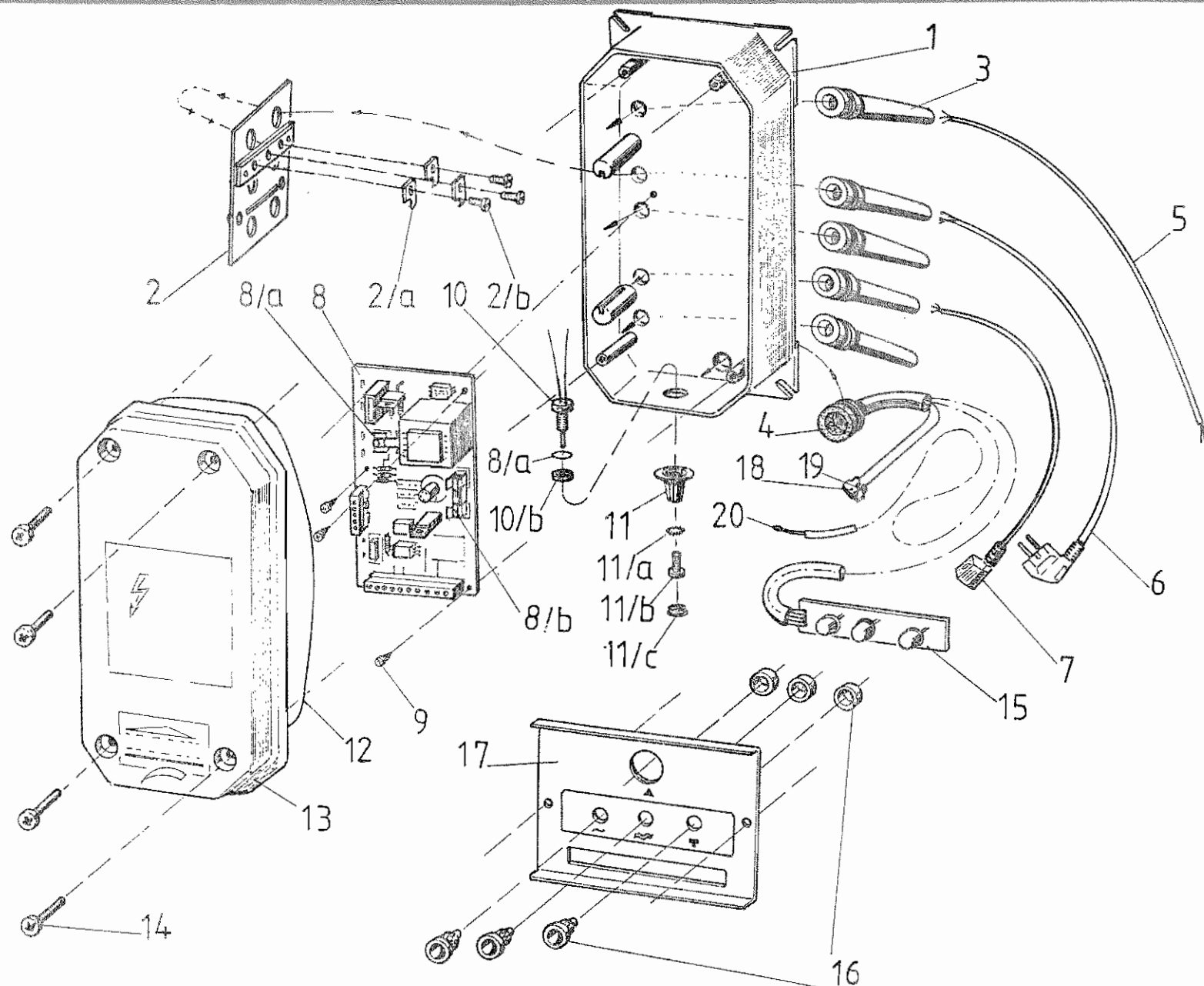
4.sz. ábra 15569-101 Szerelt elektromos egység
