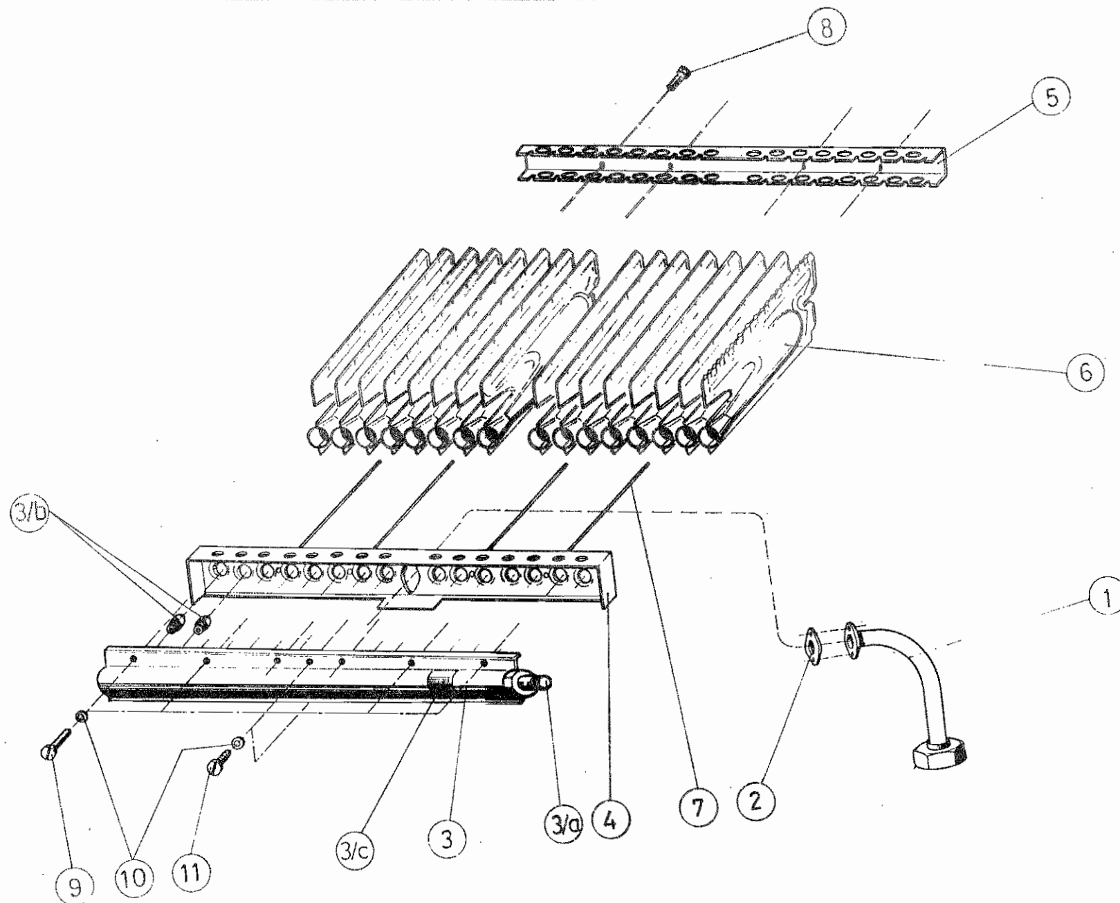
2.sz. ábra 15518-101, -102 Teljes égő
