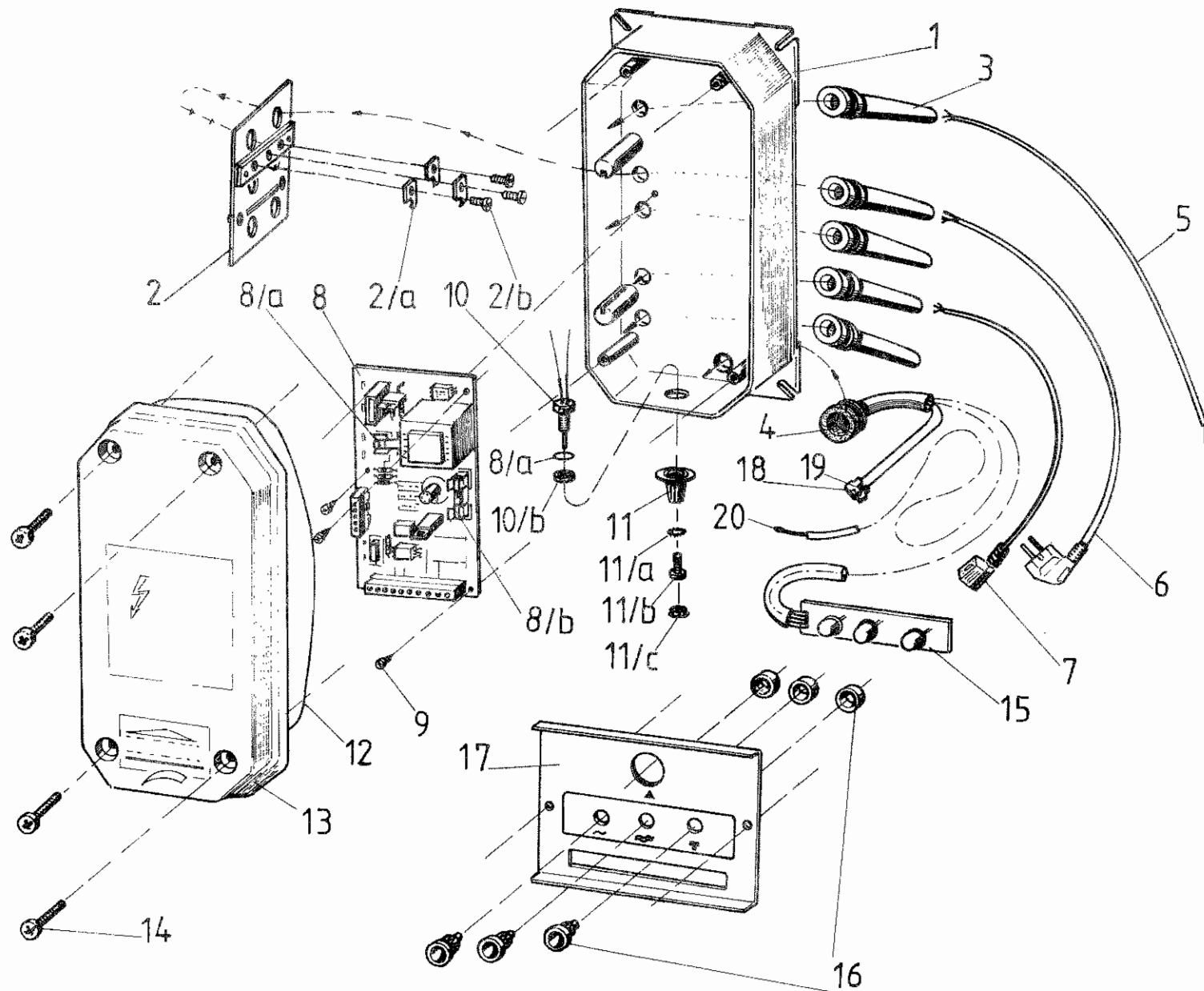
4.sz. ábra 15569-101 Szerelt elektromos egység
